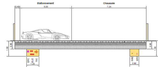
Coupe B - B
