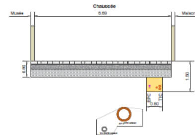
Coupe D - D
