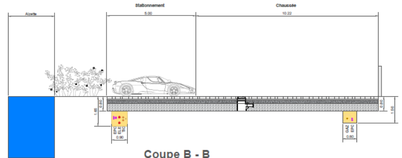
Coupe B - B
